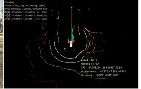
모델링한 라이다 센서의 GUI
