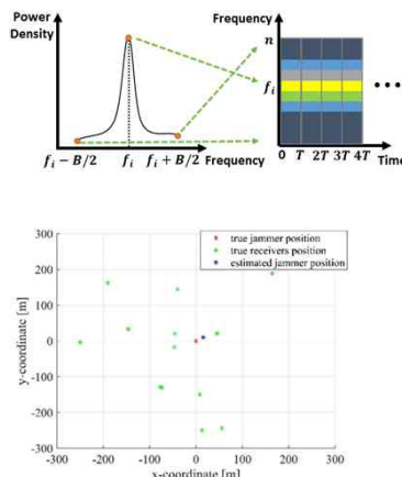
클라우드 데이터 처리방식 GNSS 재밍 감시 기술 개념도 및 시뮬레이션 결과
