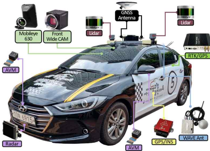
자율주행 실험 차량
