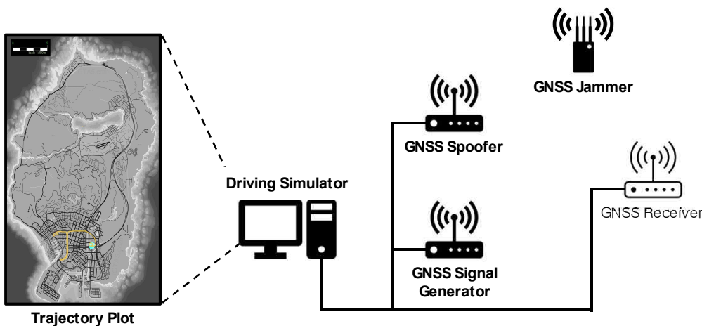
드라이빙 시뮬레이터 기반 GPS-HILS 구성도
