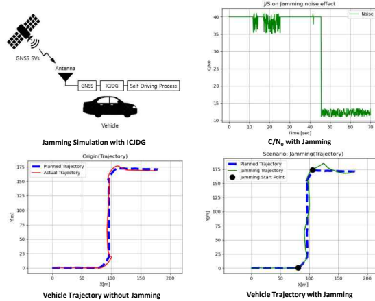
재밍 발생 시뮬레이션 환경 및 결과
