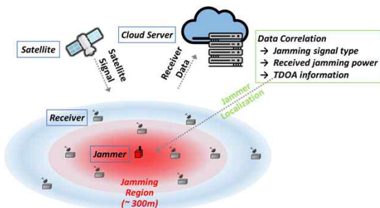
클라우드 데이터 처리방식 GNSS 재밍 감시 기술 개념도 및 시뮬레이션 결과
