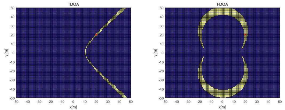
TDOA와 FDOA 기반 위치 추정
