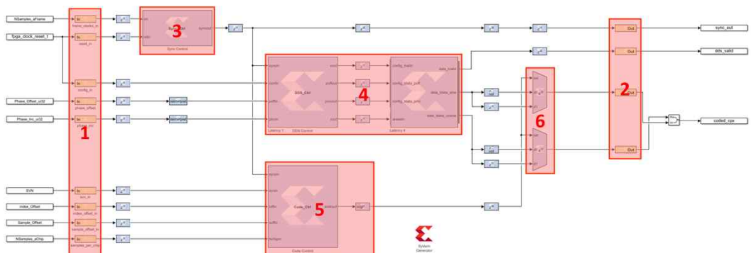
GPS L1 C/A 1채널 IF 신호 생성기 구조
